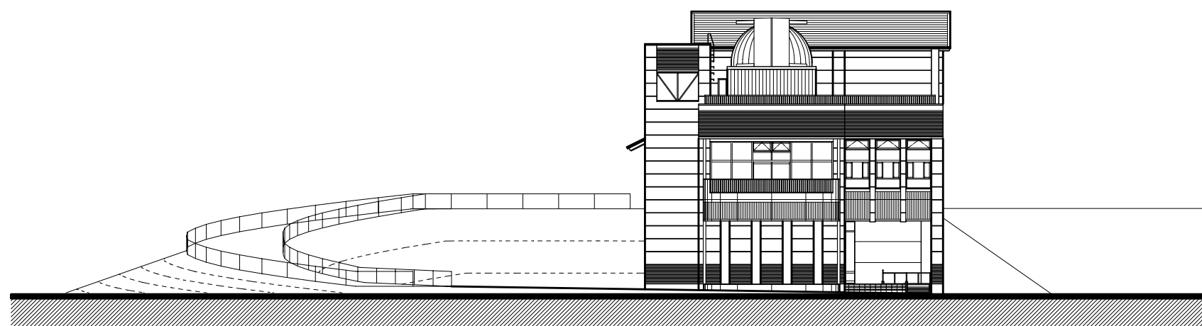
北面立面图 S = 1 / 300
