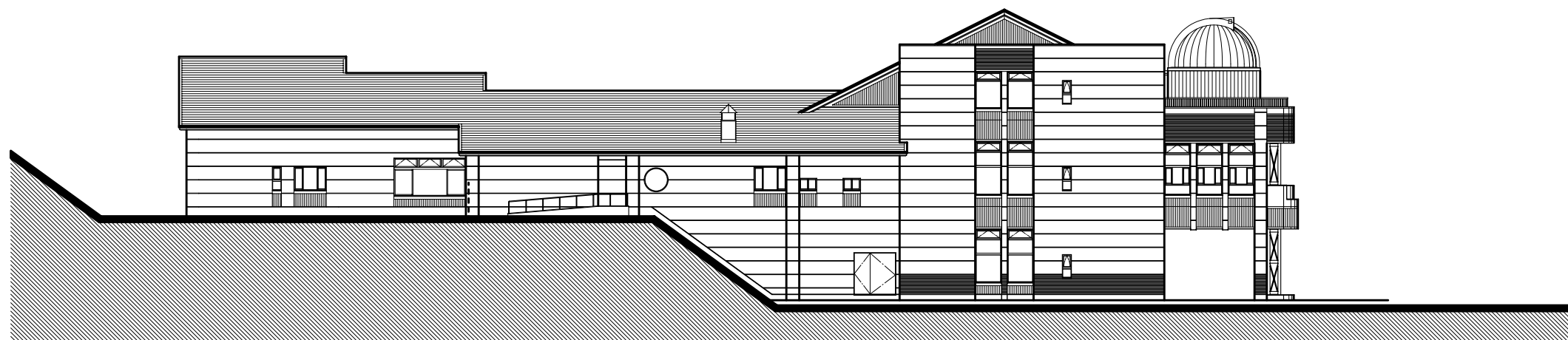
東面立面图 S = 1 / 300
