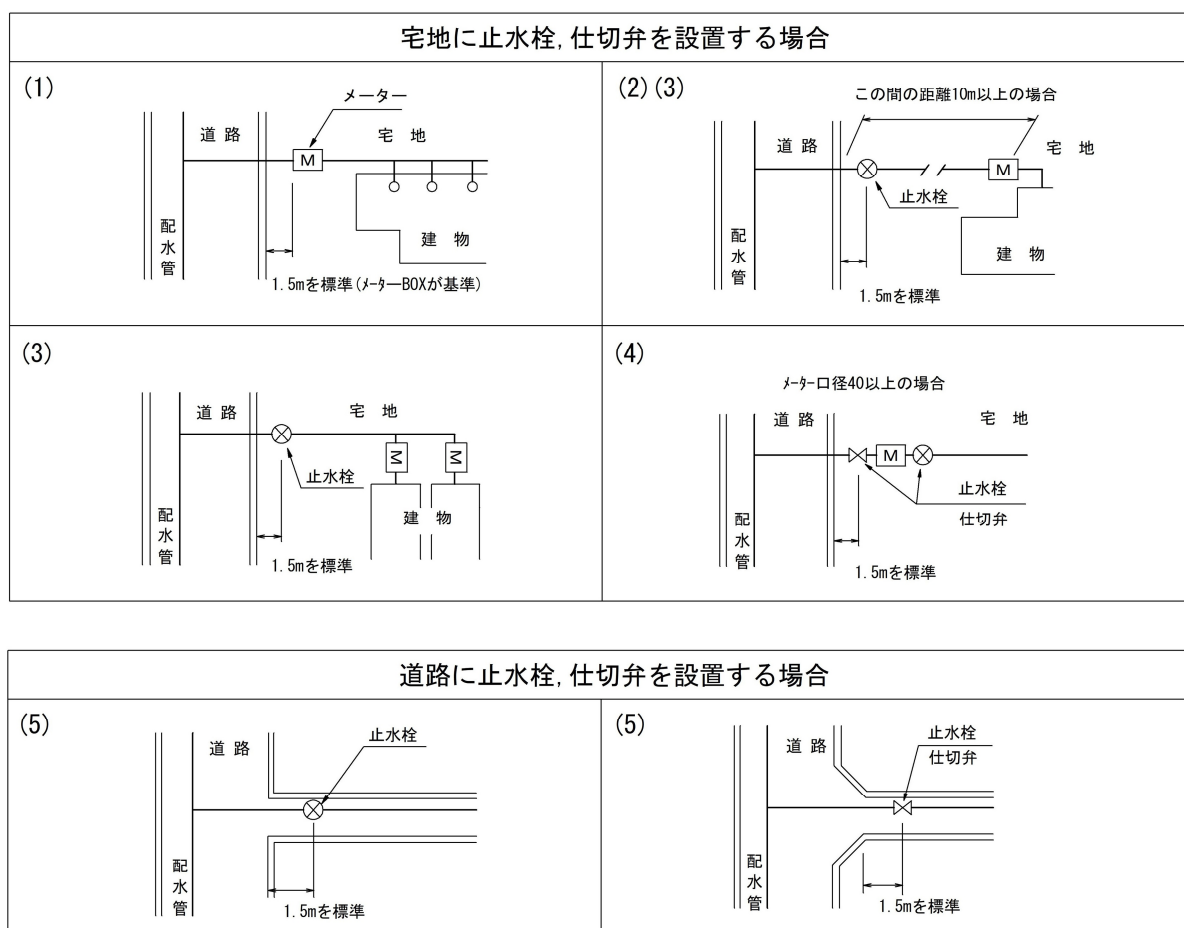
図 3-2 止水栓（仕切弁）標準設置図
