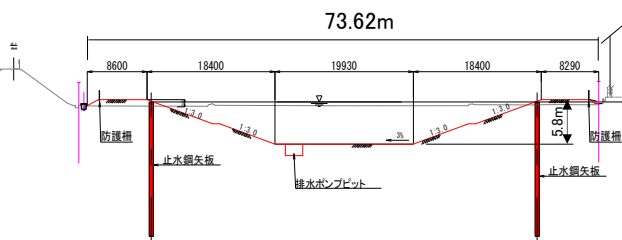
※標準断面図(計画)
