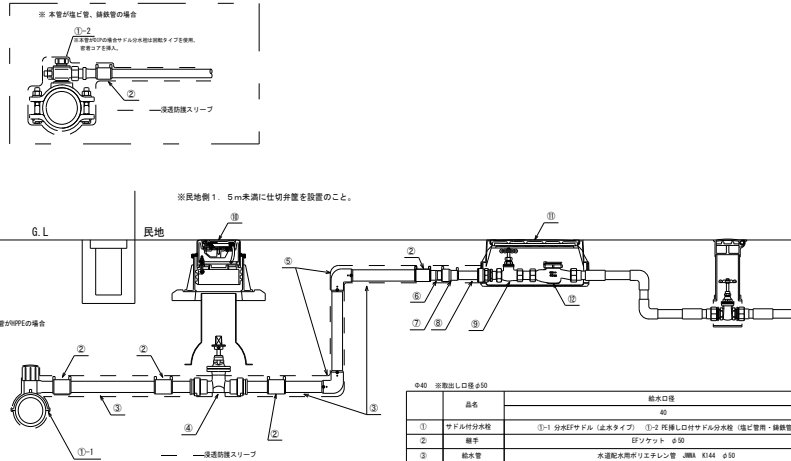
給水管標準横断面図面 (Φ40)
