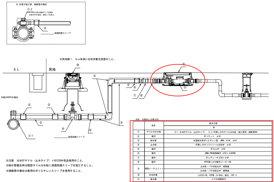
給水管標準横断面図面 (Φ40)
