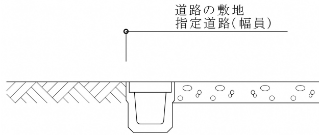
図一道路の敷地と指定道路のとり方
