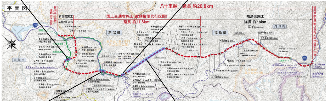
はちじゅうりごえてんくおはし 八十里越天空大橋(5号橋梁)
