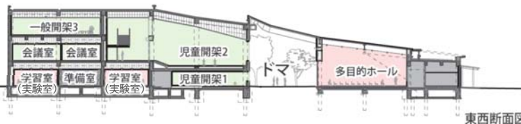
東西断面図
