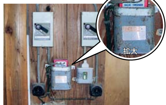
低圧進相コンデンサ
