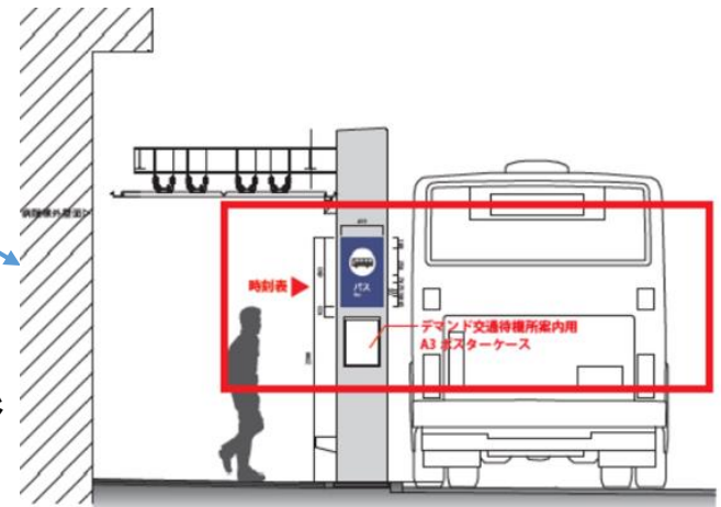
■バス停立面図 (バス停サイン側)
